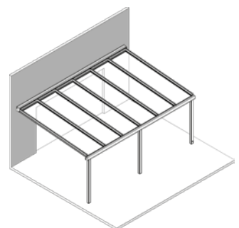
B3 Bündig, 3. Steher
