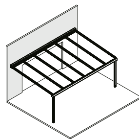
B1 Bündig, Steher außen
