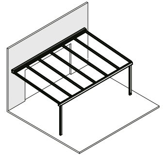
B1 Bündig, Pfosten außen
