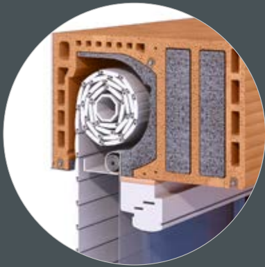
Ziegel-Rollladenkasten mit Rollladen und integriertem Insektengitter-Rollo
