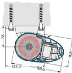
Deckenbefestigung
