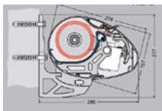
Wandbefestigung
