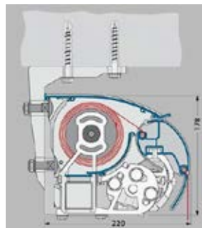
Deckenbefestigung
